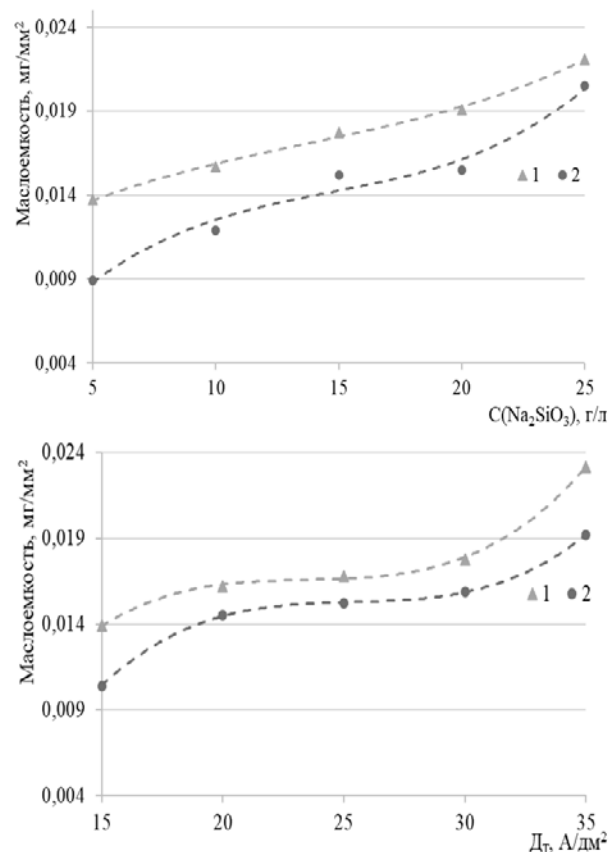
Рис. 3. Зависимость маслосъемности покрытий от (а) концентрации \text{Na}_2\text{SiO}_3 в электролите ( T = 1,5 часа; \text{СКОН} = 2 г/л, \text{ДТ} = 25 А/дм 2 ) и (б) от плотности тока ( T = 90 мин, \text{СКОН} = 2 г/л, \text{CNa}_2\text{SiO}_3 = 15 г/л): 1 – сплав АК7ч; 2 – сплав АО3-7
